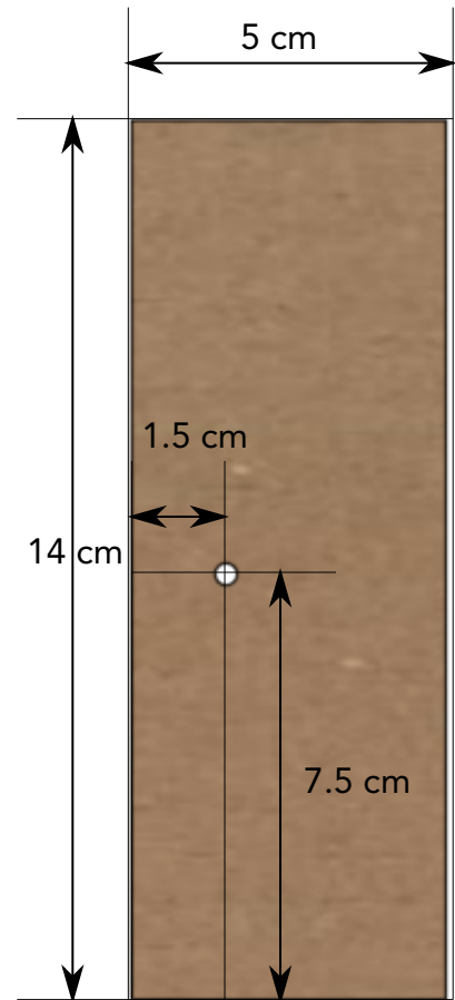
SIDEWALL (x2)
